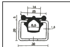
Ruban isolant en caoutchouc type RU 25
